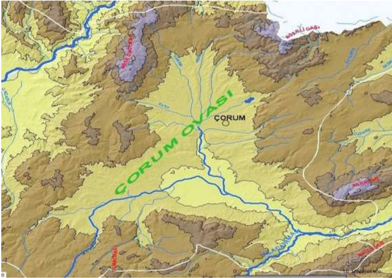
Şekil 5: Çorum Ovası ve çevresinin topografya haritası (Yeşilirmak Havzası Coğrafi Bilgi Sistemlerinden alınmıştır).
