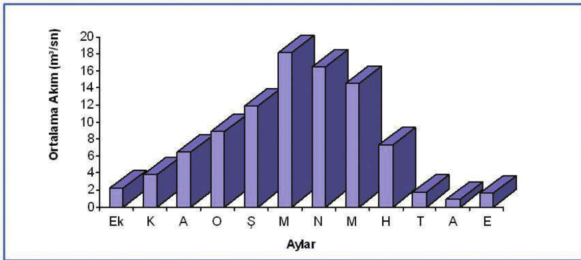
Şekil 12: Çorum Çayının akım diyagramı. (Şeyhoğlu Hidrometri İstasyonu, 1962-1990)
