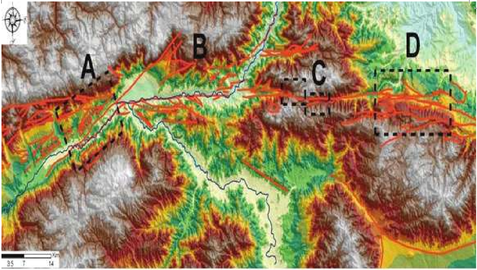
Şekil 9: İnceleme alanının aktif fayları ve üç boyutlu morfolojik haritası. A bölgesi Tosya-Oğuz ve Devrez Faylarını, B bölgesi Kargı Ovası ve Kızılırmak Fayını, C ve D bölgesi ise Kızılırmak-Köprübaşı Faylarını göstermektedir. Kareler detaylı şekillerin yerleridir.
